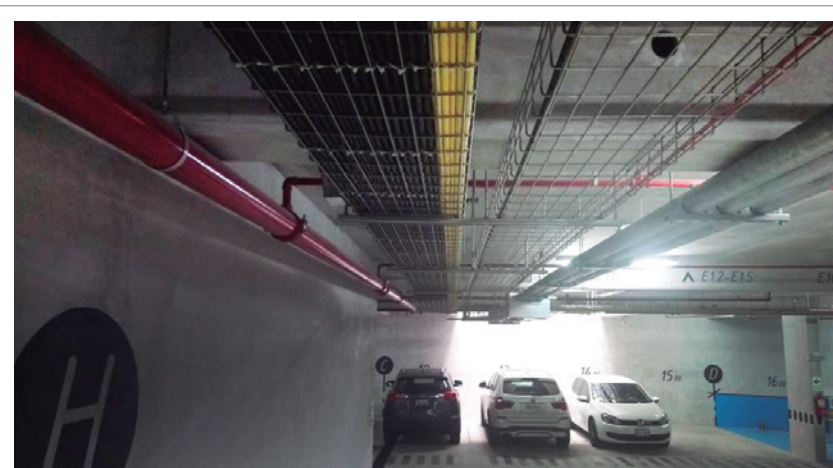
Bandejas tipo Rejilla "Viafil" en Playa de Estacionamiento - San Isidro
