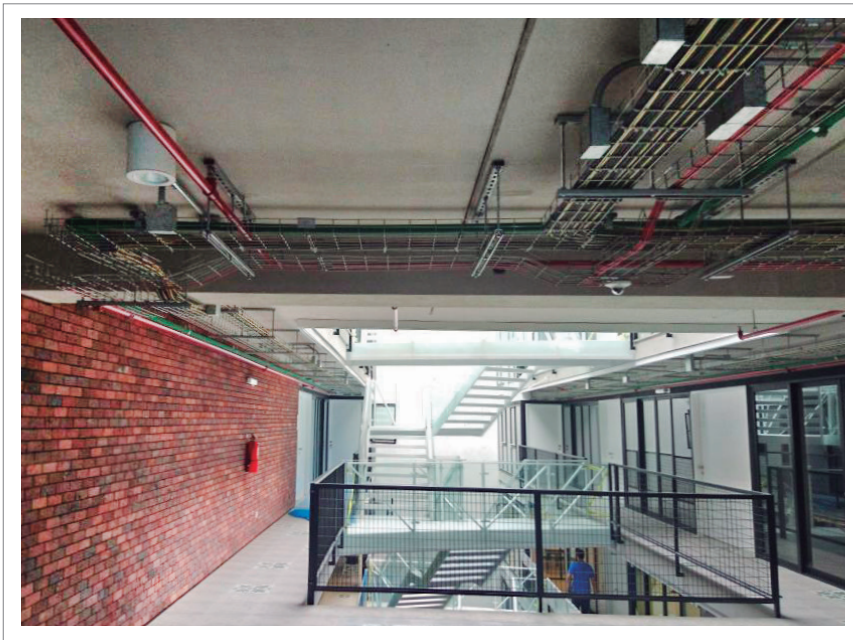
Bandejas tipo Rejilla "Viafil" - Barranco
